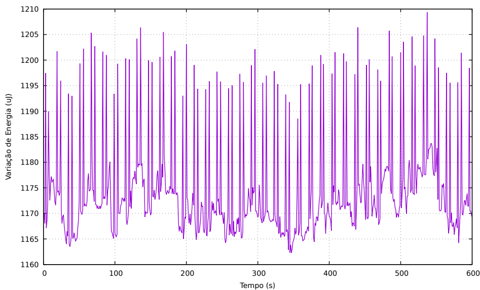
Figura 2. Teste da tarefa ociosa
