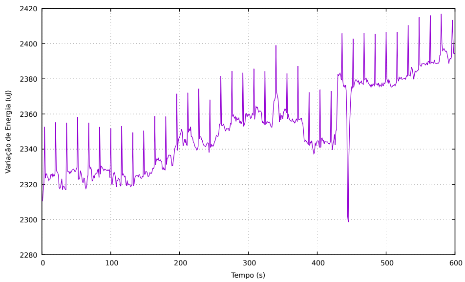
Figura 4. Teste da tarefa Housekeeping
