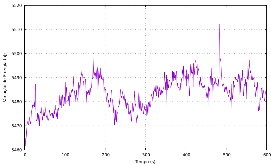
Figura 5. Teste da tarefa Communications
