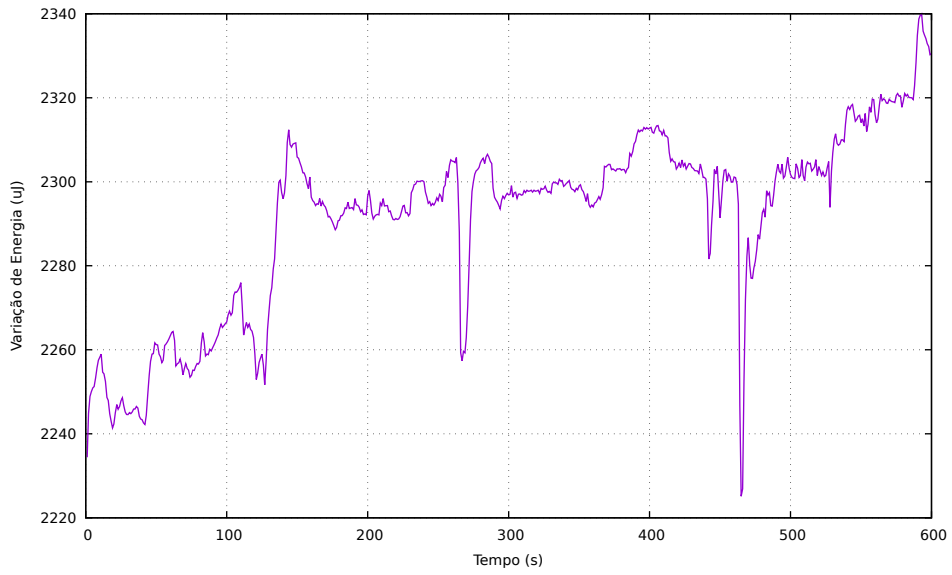
Figura 3. Teste da tarefa Watchdog
