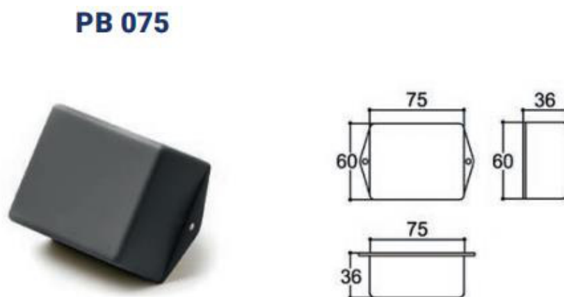
Figura 4 - Caixa patola PB-075
