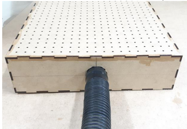
Figura 14 - Caixa termoformadora conectada ao aspirador de pó
