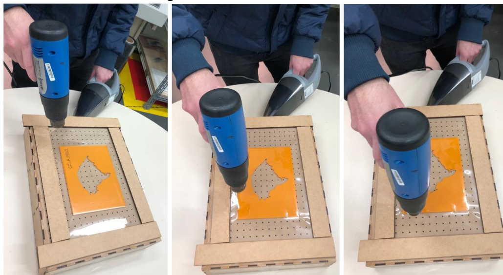
Figura 23 - Termoformadora em uso
