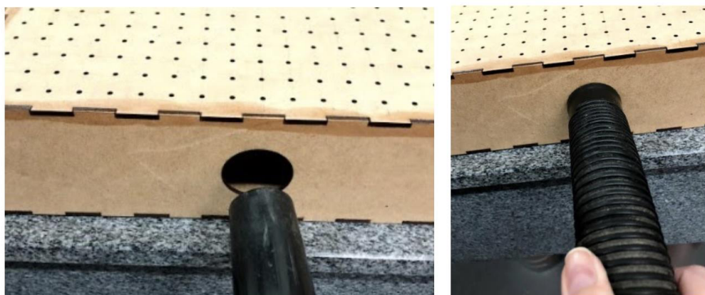
Figura 21 - Bocal do aspirador de pó encaixado no furo lateral
