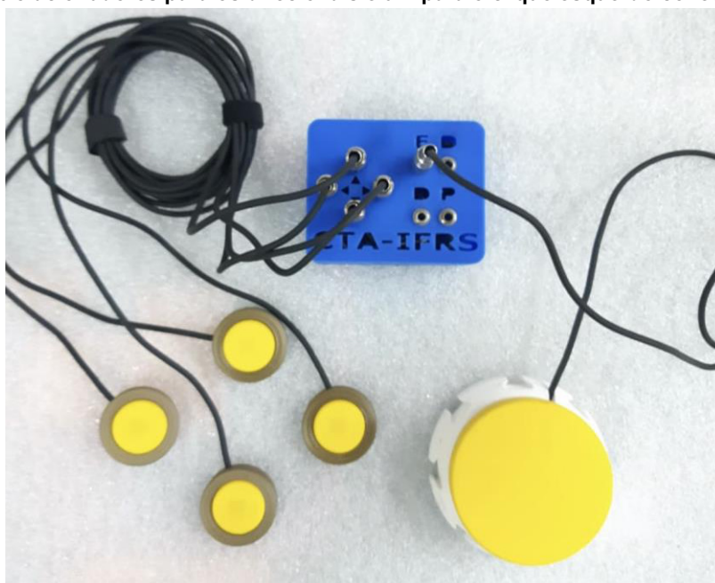
Figura 19 - Quatro acionadores para os direcionais e um para o clique esquerdo conectados ao mouse
