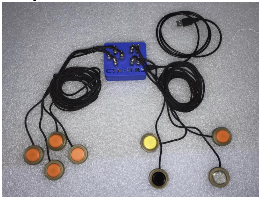
Figura 18 - Oito acionadores conectados ao mouse com Arduino
