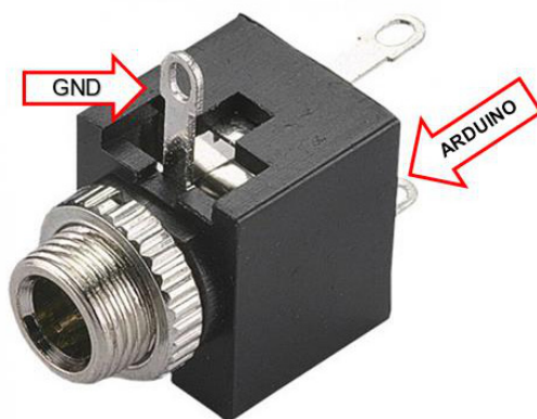
Figura 14 - Indicação dos pinos de ligação do Jack J2
